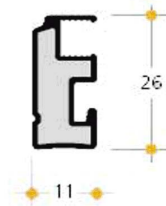
Dimension du profilé
